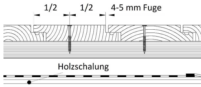
Bild 2. Befestigung mittig auf der sichtbaren Brettbreite
