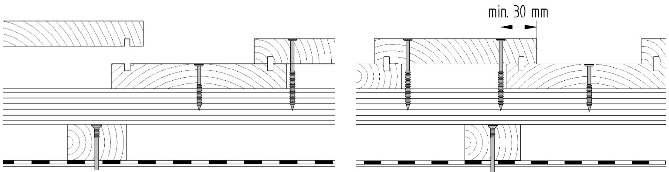
Bild 3. Befestigung unteres Dachprofil
