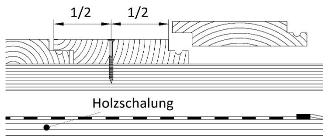
Bild 1. Verlegung mit der Hohlkehle nach Oben
