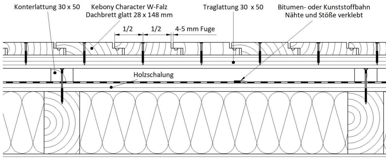
Regensicheres Unterdach mit Belüftung
